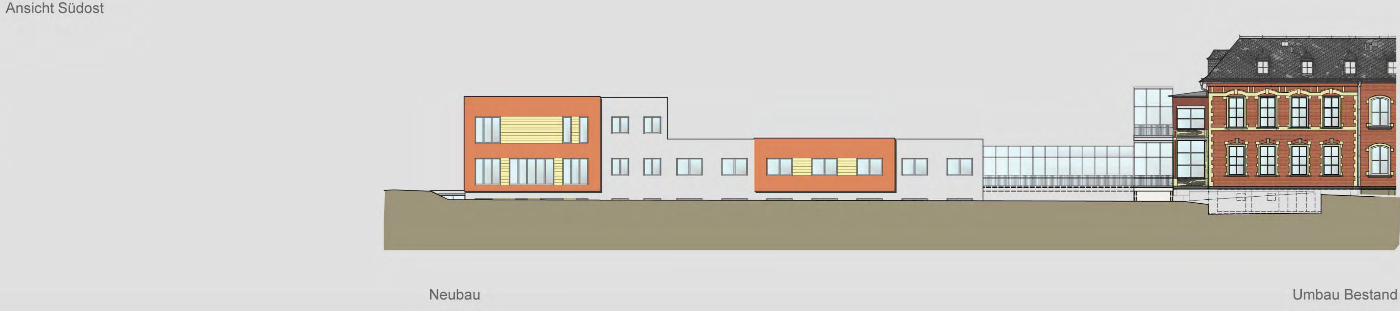
Ansicht Südost
