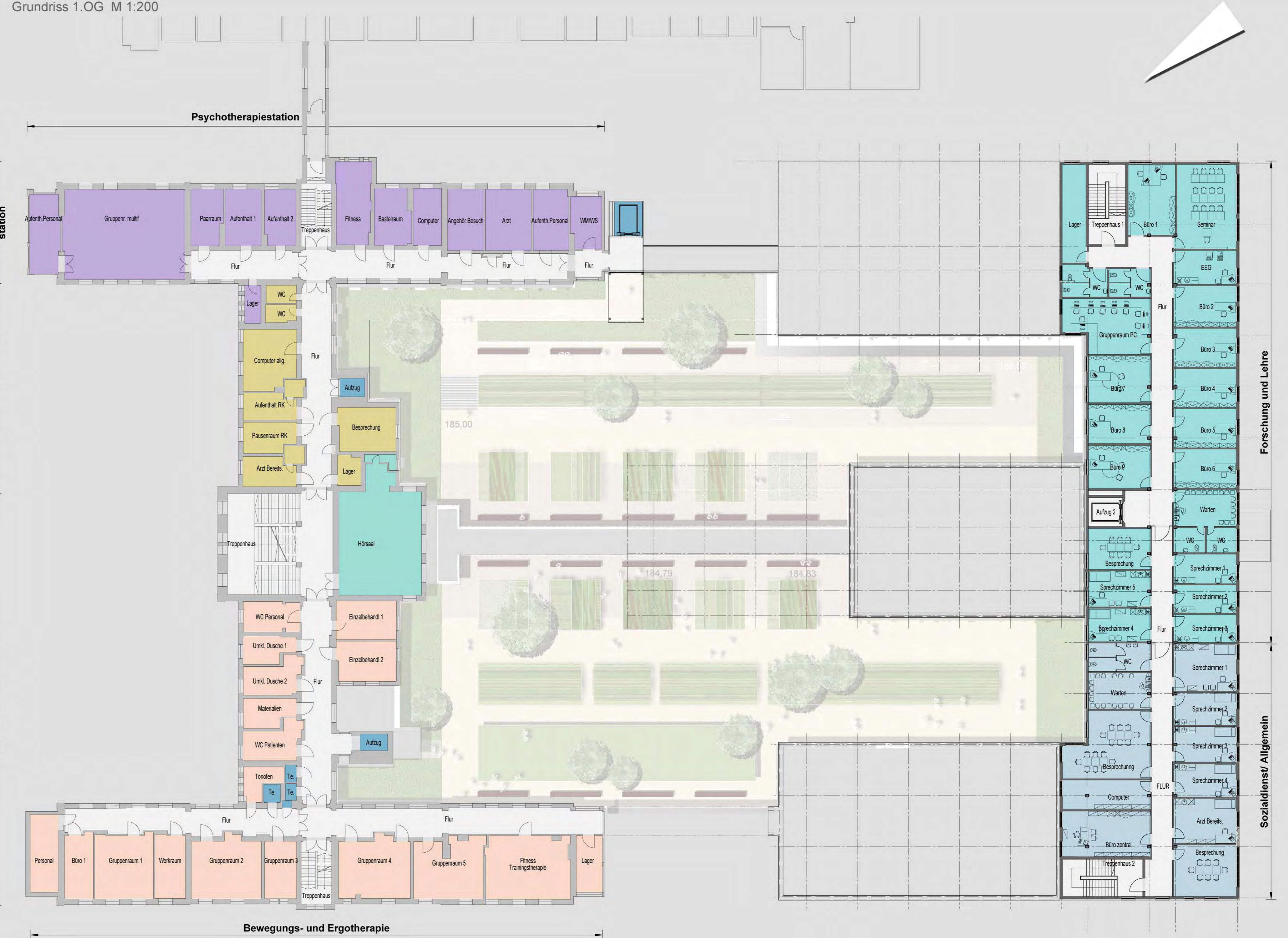
Grundriss 1.OG M 1:200
