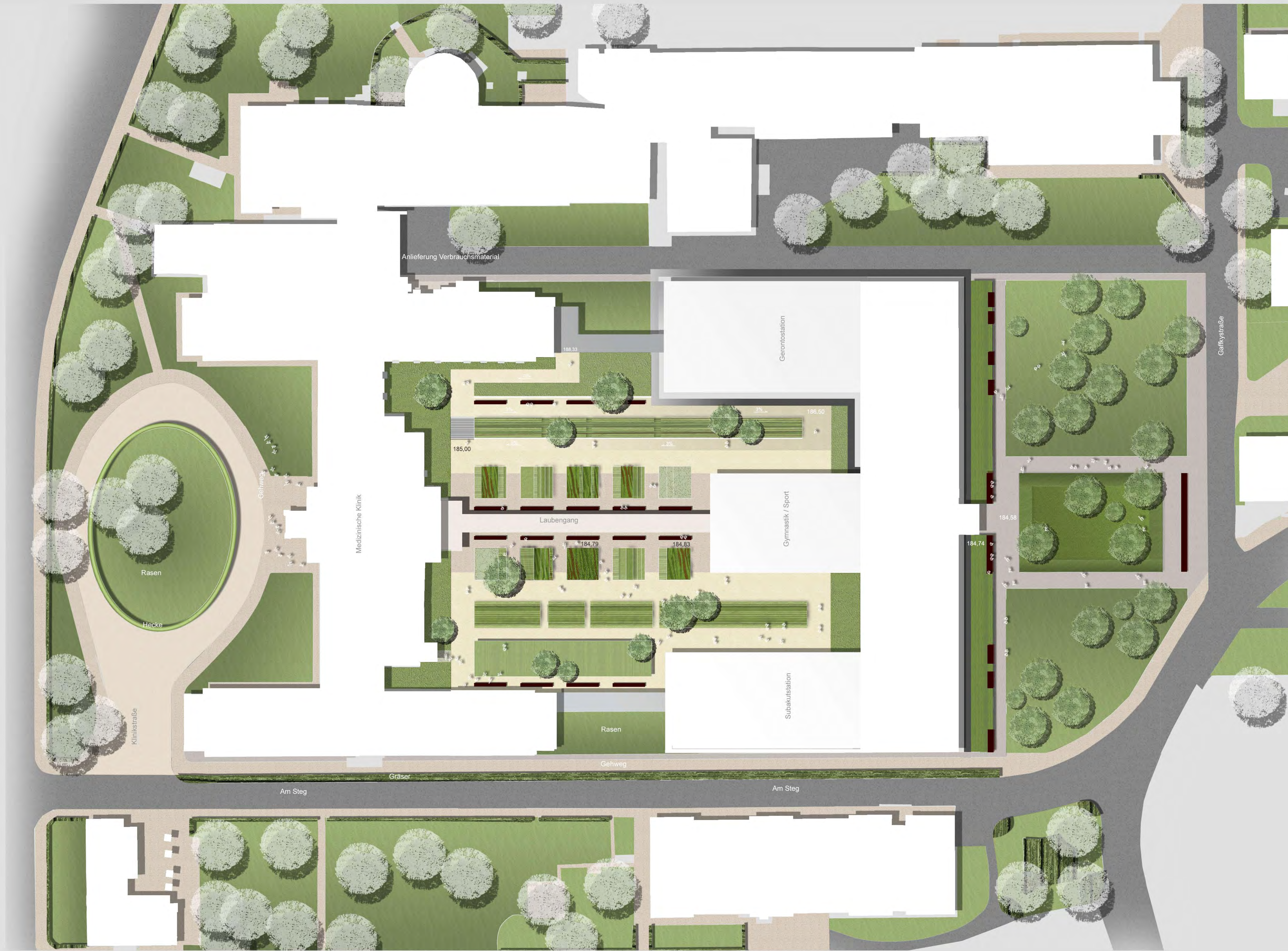
Lageplan M 1:250
