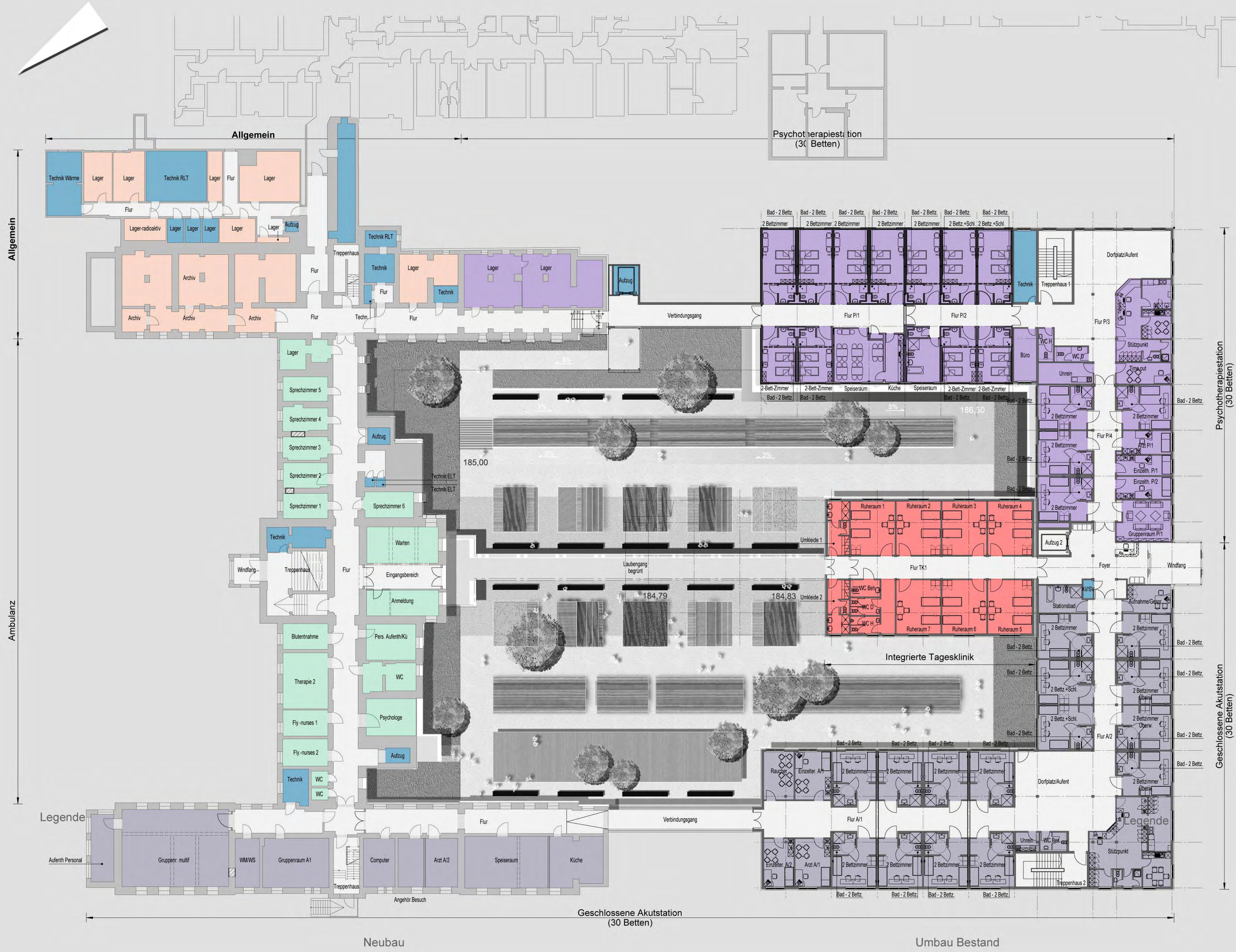
Grundriss KG M 1:200
