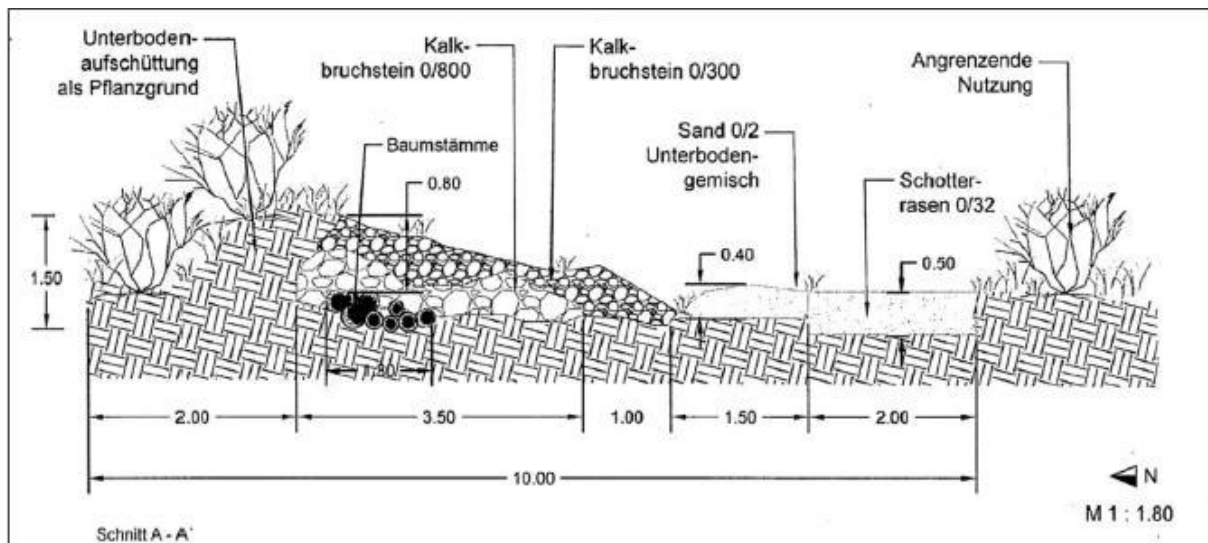
Abbildung 1: Schematischer Aufbau eines Steinriegelkomplexes mit Winterquartier mit Verwaltung und integriertem Eiablagesubstrat. Als Winterquartier dienen frostfrei eingebaute Totholzelemente (Quelle: Dr. Jochen Karl 2019).
