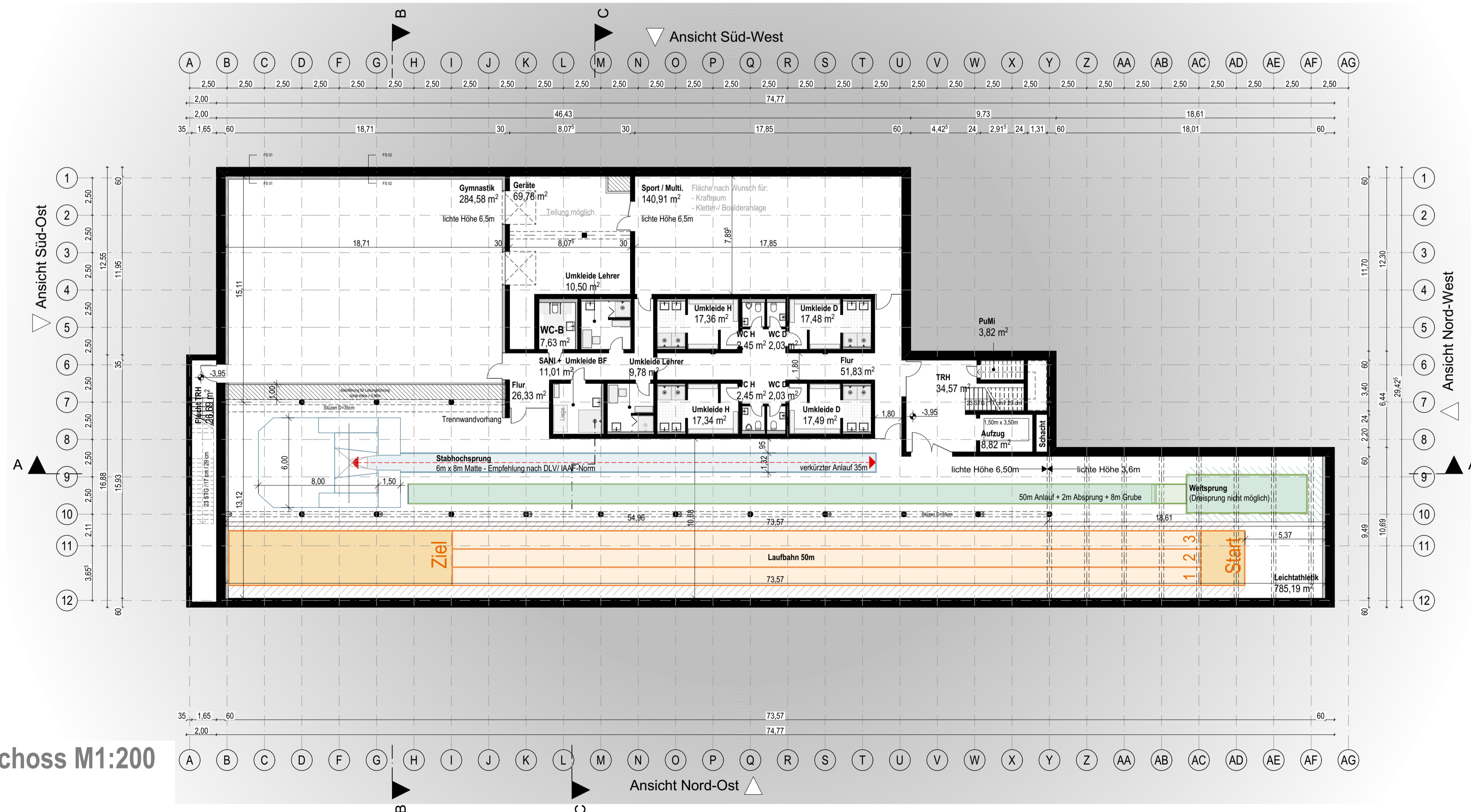
Grundriss Erdgeschoss M1:200
