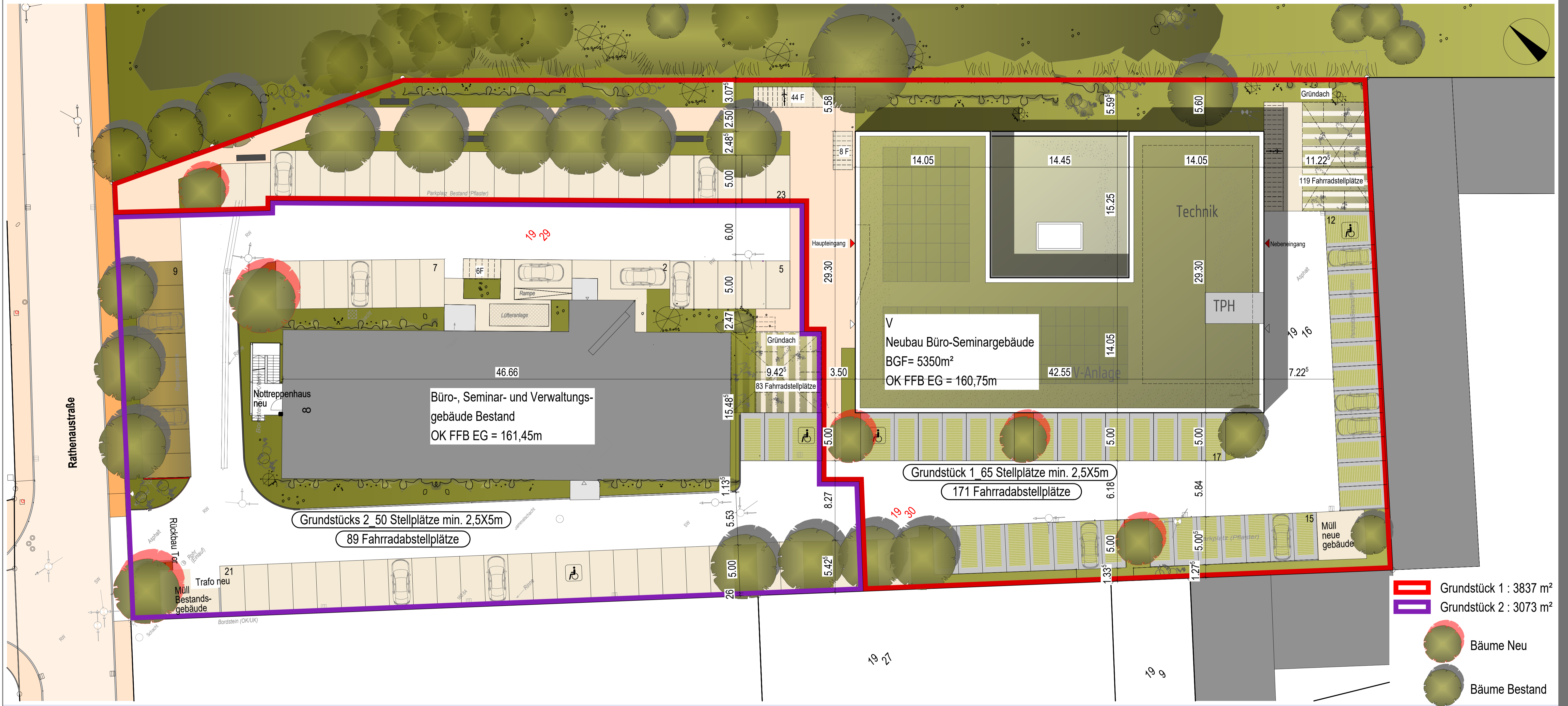
Freiflächenplan_Entwurf_04a_M200
