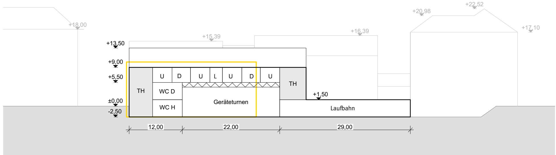
Schnitt A-A
