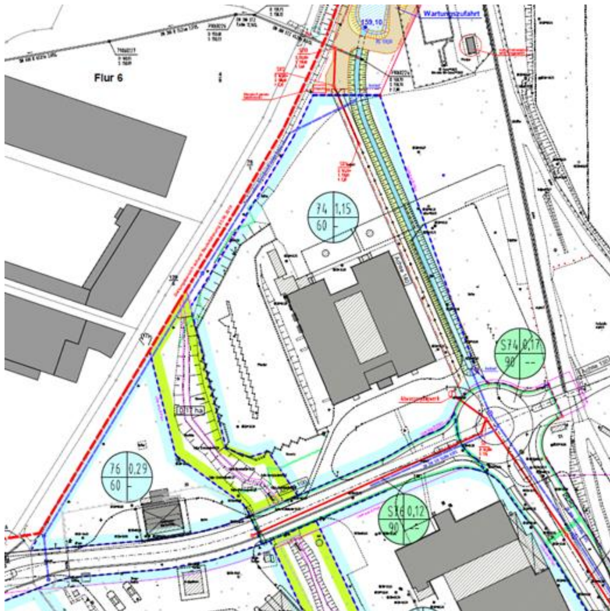
Vorabzug Vorentwurf Lageplan Entwässerung , Büro HS Ingenieure, 06/2019
