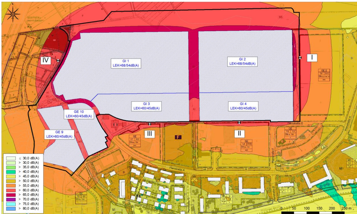
Lärmkarte der Beurteilungspegel (erhöhter Ansatz; korrigiert/reduziert, s.o.)
