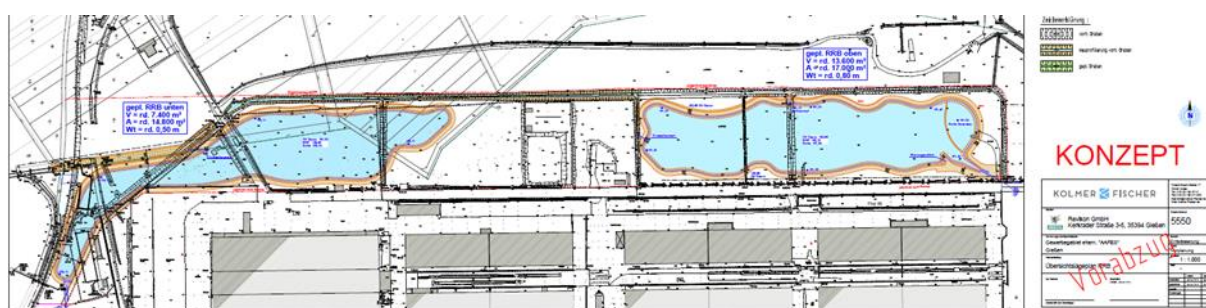
Vorplanung Entwässerung Lage Regenrückhaltebecken, Büro HS-Ingenieure, 01/2019
