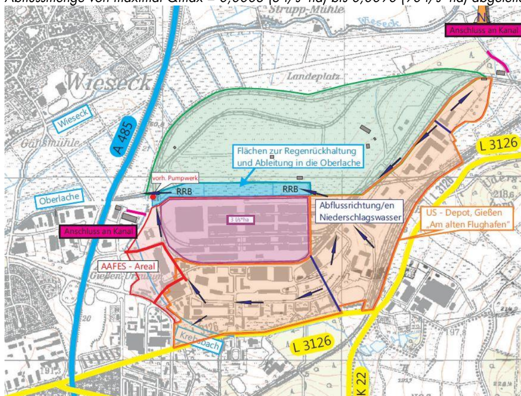
Entwässerungsplanung HS-Ingenieure, 2019
