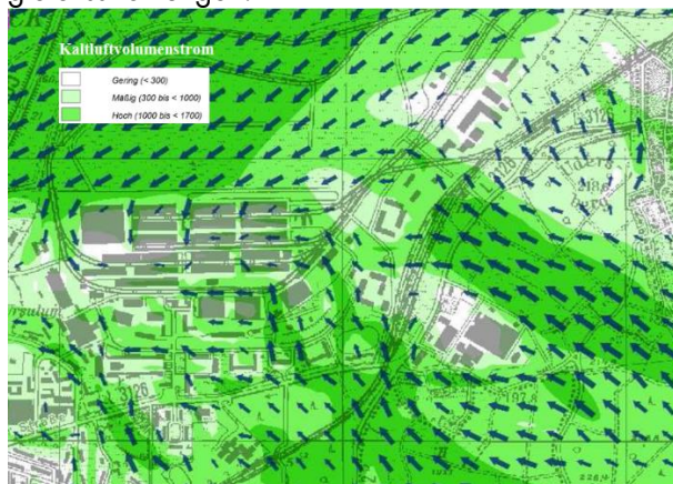
Ausschnitt Detailkarte Kaltluftvolumenstrom
