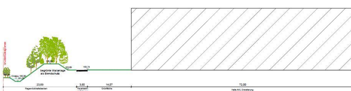
Geländeschnitt mit bepflanzter Wallanlage und naturnaher Regenrückhaltung (Anpflanzfläche A3)
