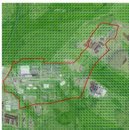
Das bodennahe Strömungsfeld (Pfeile) und der Kaltluftvolumenstrom (Farbe) heben die Bedeutung der Planfläche als Durchtrittsbe- reich für Kaltluftströmungen Richtung Wie- seckau hervor.
