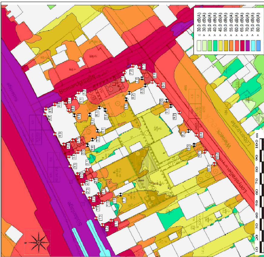
Abb. 1 : Lärmkarte der Beurteilungspegel
