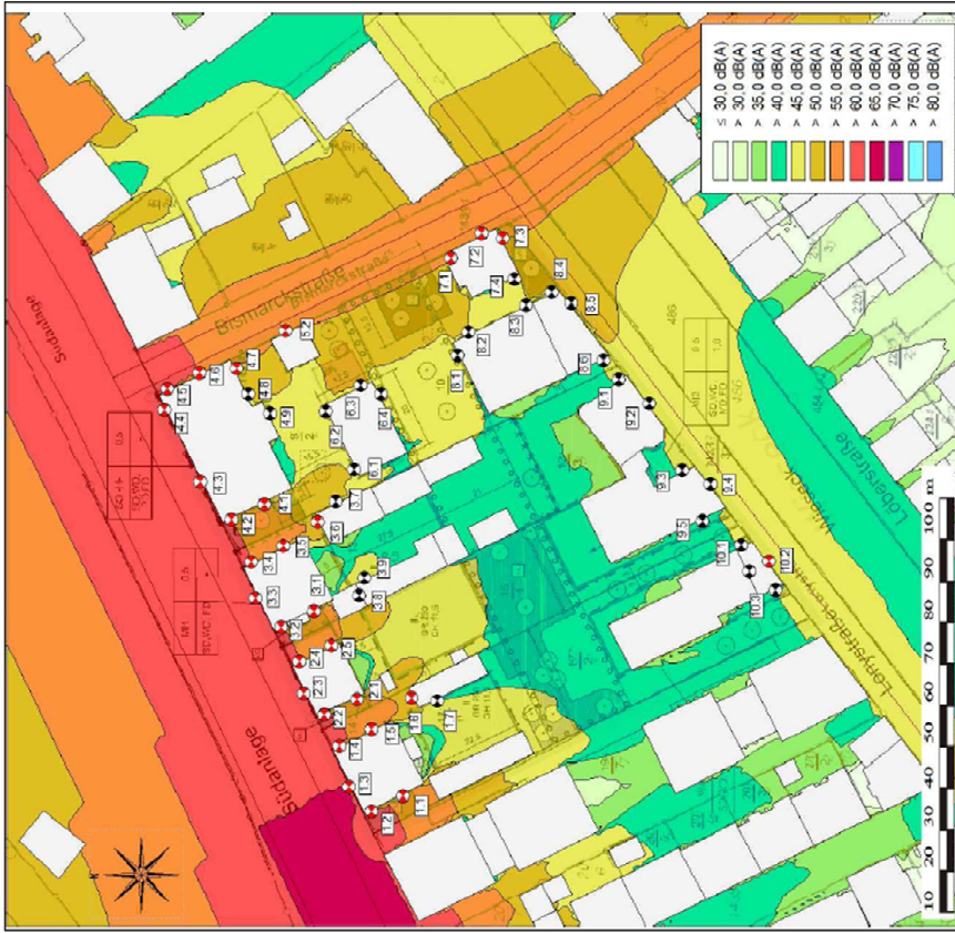
Abb. 4 : Lärmkarte der Beurteilungspegel - Nachtzeit - Höhe 1. Obergeschoß.
