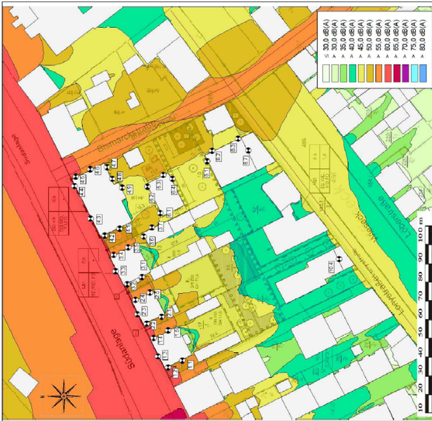
Abb. 6 : Lärmkarte der Beurteilungspegel - Nachtzeit - Höhe 2. Obergeschob.
