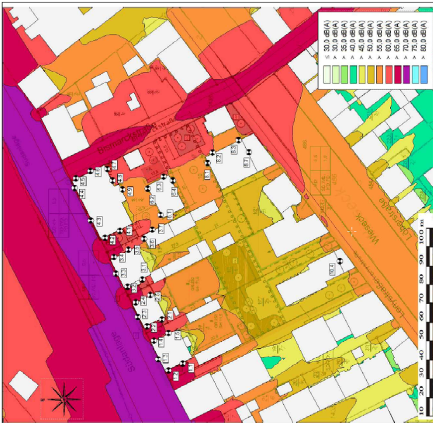
Abb. 5 : Lärmkarte der Beurteilungspegel - Tagzeit - Höhe 2. Obergeschob.
