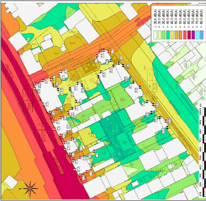
Abb. 2 : Lärmkarte der Beurteilungspegel
