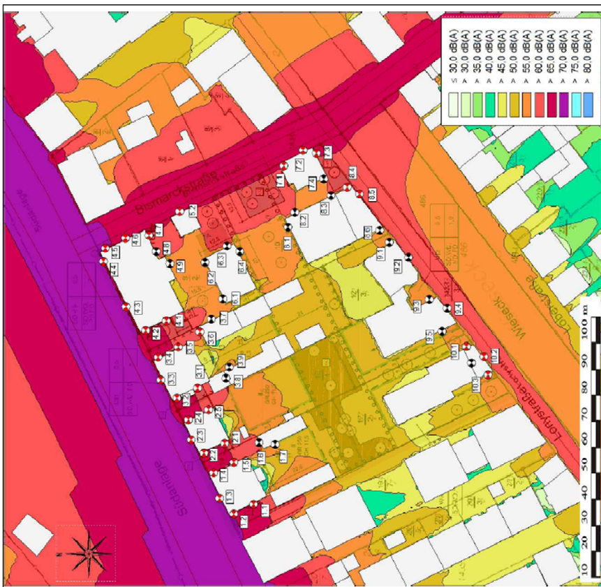
Abb. 3 : Lärmkarte der Beurteilungspegel - Tagzeit - Höhe 1. Obergeschoß.
