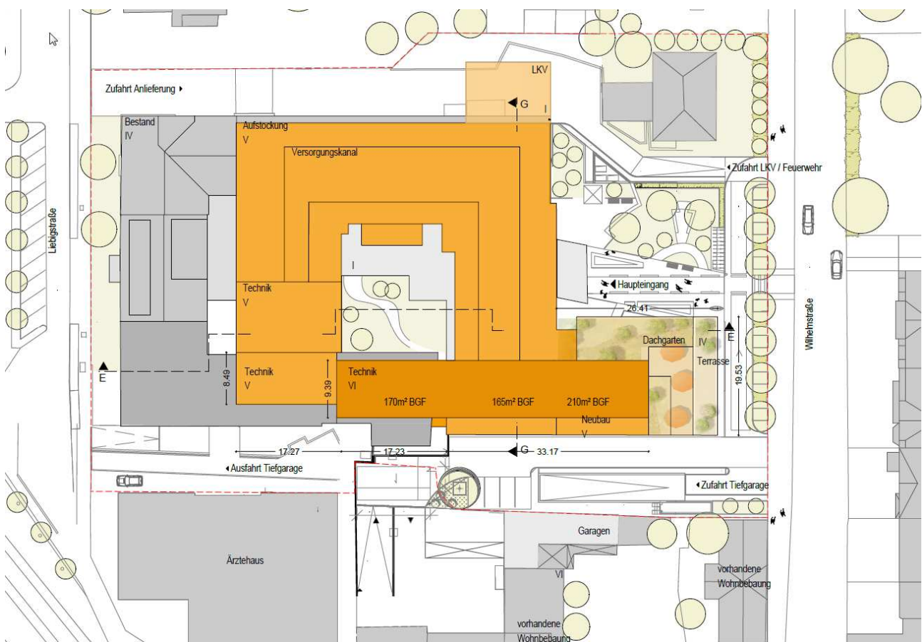
Lageplan mit Darstellung der baulichen Änderungen (orange), sander.hofrichter architekten GmbH | Gesellschaft für Architektur und Generalplanung, Plot-Datum 25.01.2018
