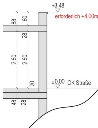
Systemschnitt eingeschossig erforderliche Höhen
