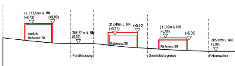
Schnitt 1
