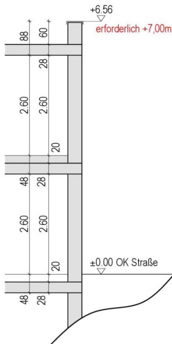
Systemschnitt zweigeschossig erforderliche Höhen
