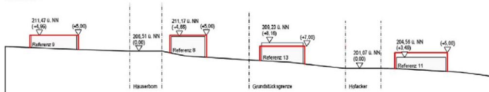
Schnitt 2
