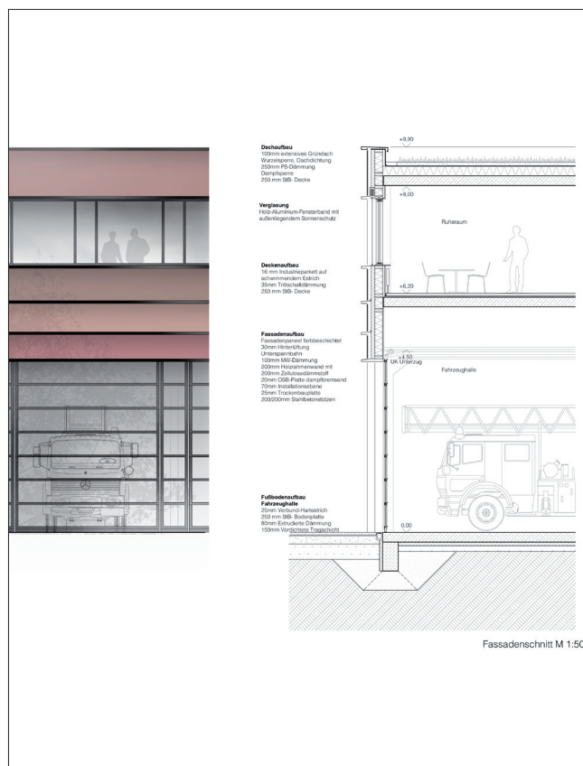
Vertiefung Fahrzeughalle
